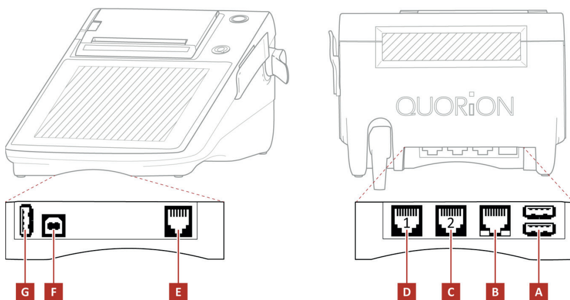
Abbildung 4: Übersicht Schnittstellen
